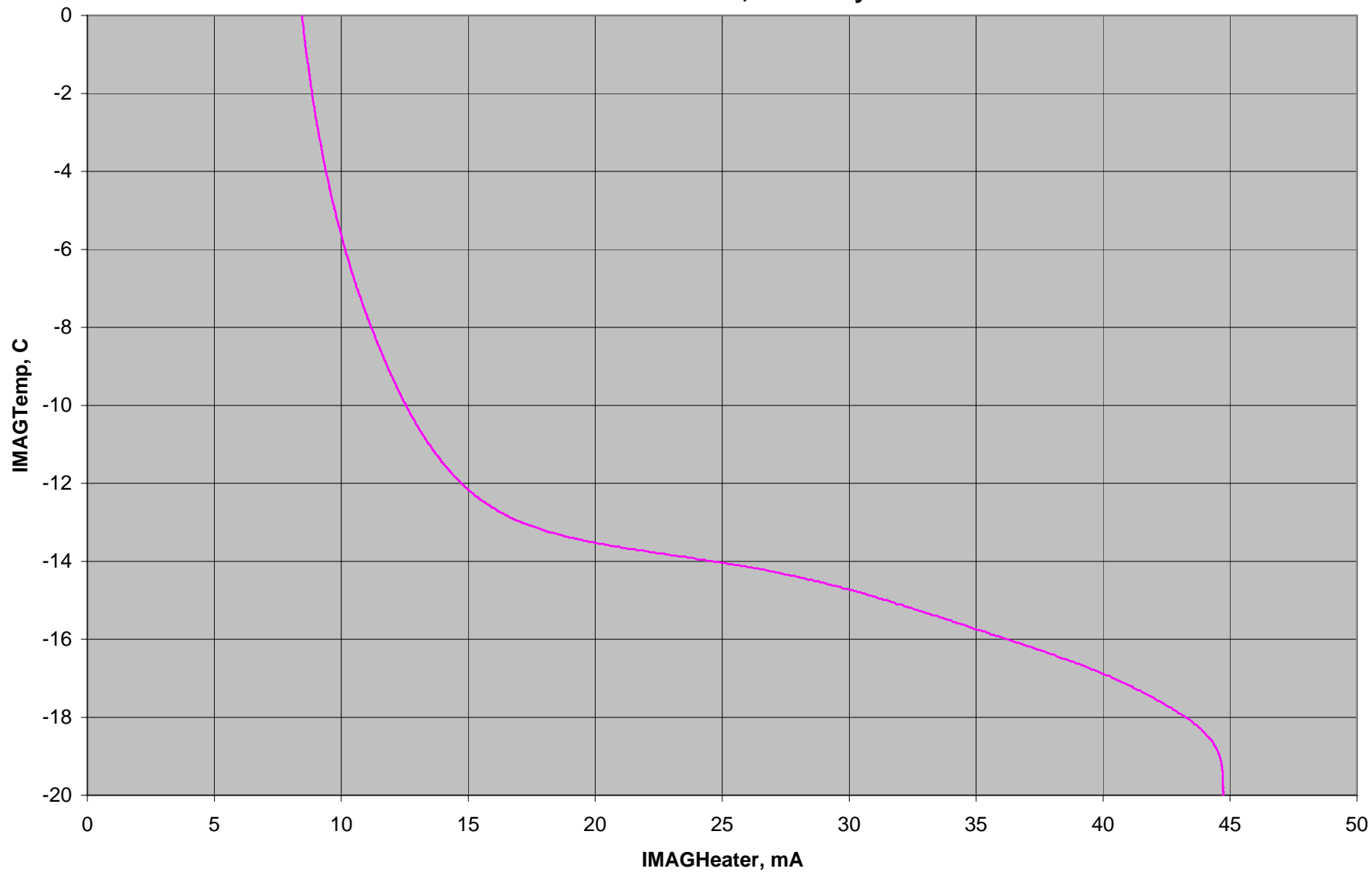
FM1 MAG Thermal Vac, 2004-July-7
